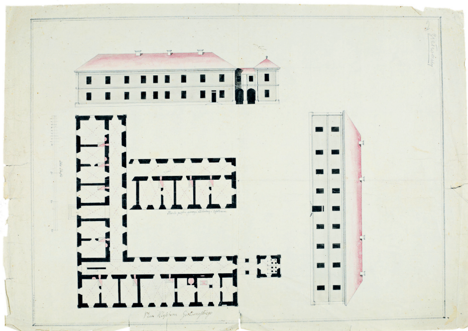
Il. 1. Plan i fasada klasztoru gielwańskiego (lit. Gelvonai), 1788 r., architekt K. Kamiński; VUB RS, F73-294, k. 1.
