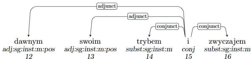
Rysunek 5. Fragment drzewa zależności składniowych zawierający pary dawnym trybem i swoim trybem
