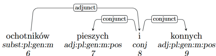
Rysunek 4. Fragment drzewa zależności składniowych zawierający pary ochotników pieszych i ochotników konnych
