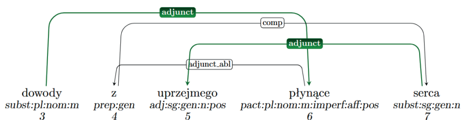
Rysunek 7. Pary dowody płynące i uprzejmego serca
