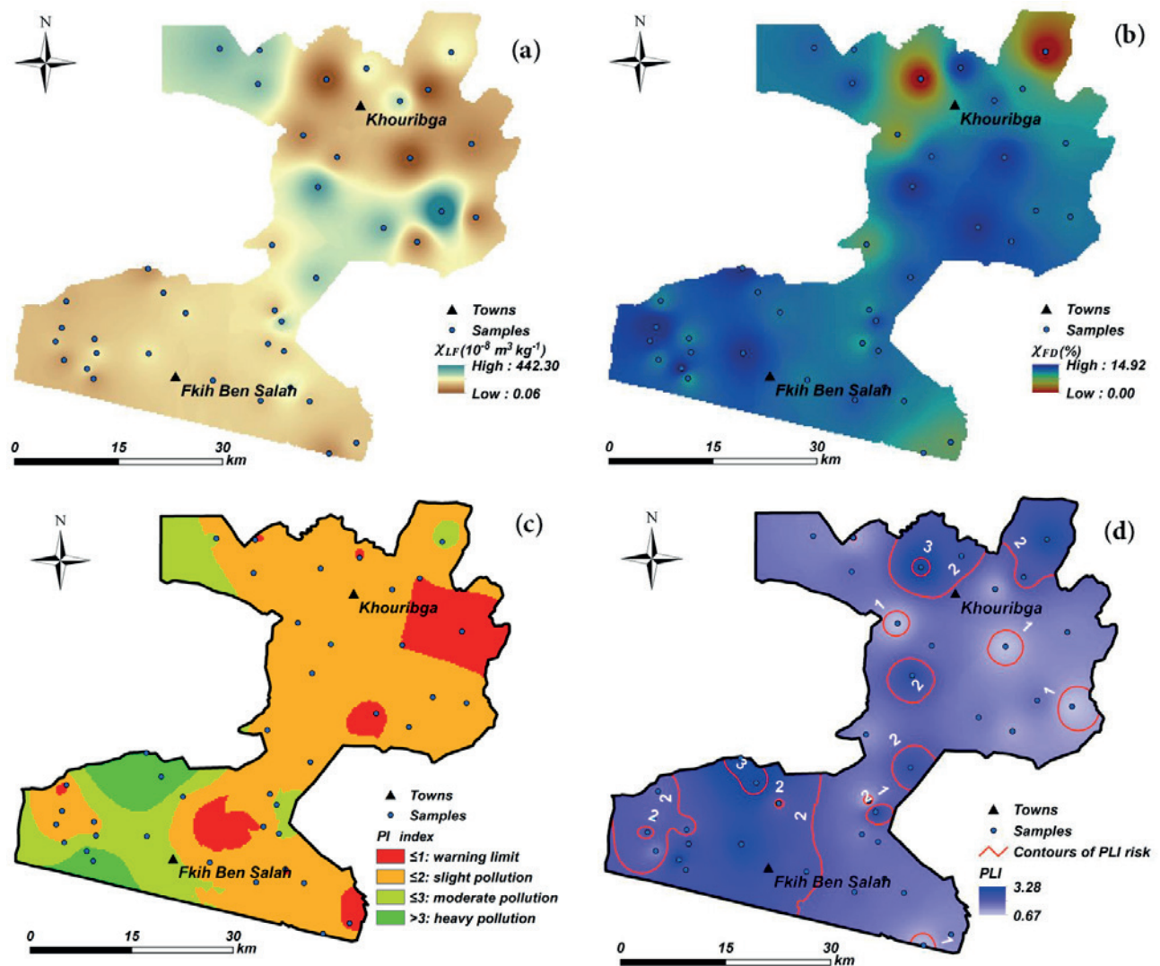
Figure 3. Maps of values of \chi_{LF} (a), \chi_{FD} (b), PI (c) and PLI (d)
