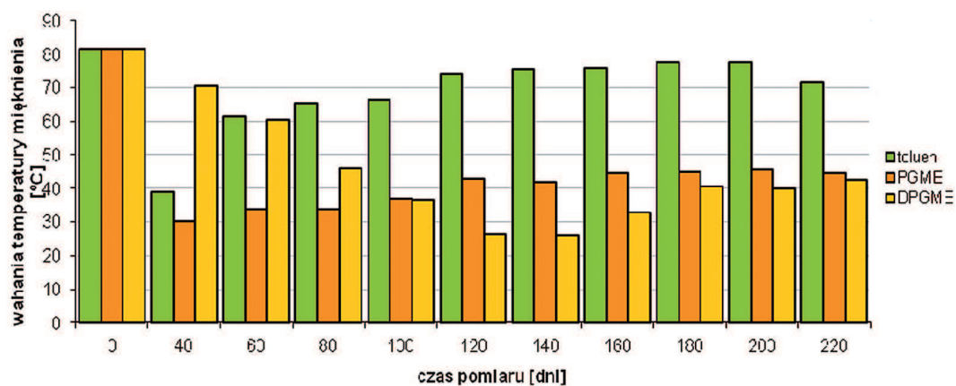
Wykres 5. Wyniki pomiarów zmian temperatury mięknięcia warstw polichromii deski ze stopni schodów ambony, w rezultacie przeprowadzonego zabiegu impregnacji 10% roztworami Paraloidu B-72 w toluenie, 1-metoksy-2-propanolu i eterze metylowym glikolu dipropylenowego 45
