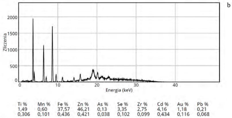
Il. 16. Morąg, kościół św. Apostołów Piotra i Pawła. Prezbiterium, fragment ściany północnej, malowidło Wielka Rodzina Marii . Wyk. J. Raczkowski a – pomiar 4, b – widmo XRF
