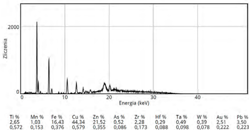
Il. 18. Morąg, kościół św. Apostołów Piotra i Pawła. Prezbiterium, fragment ściany północnej, malowidło Wielka Rodzina Marii . Wyk. J. Raczkowski a – pomiar 6, b – widmo XRF
