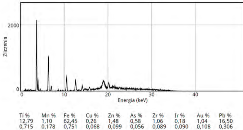
Il. 17. Morąg, kościół św. Apostołów Piotra i Pawła. Prezbiterium, fragment ściany północnej, malowidło Wielka Rodzina Marii . Wyk. J. Raczkowski a – pomiar 5, b – widmo XRF
