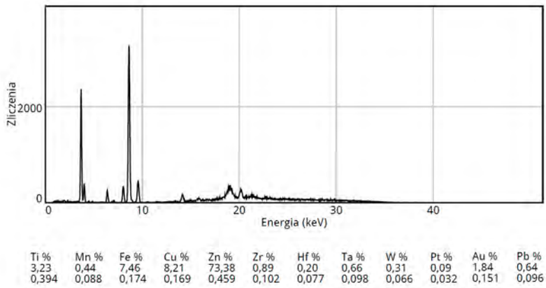
Il. 19. Morąg, kościół św. Apostołów Piotra i Pawła. Prezbiterium, fragment ściany północnej, malowidło Wielka Rodzina Marii . Wyk. J. Raczkowski a – pomiar 7, b – widmo XRF
