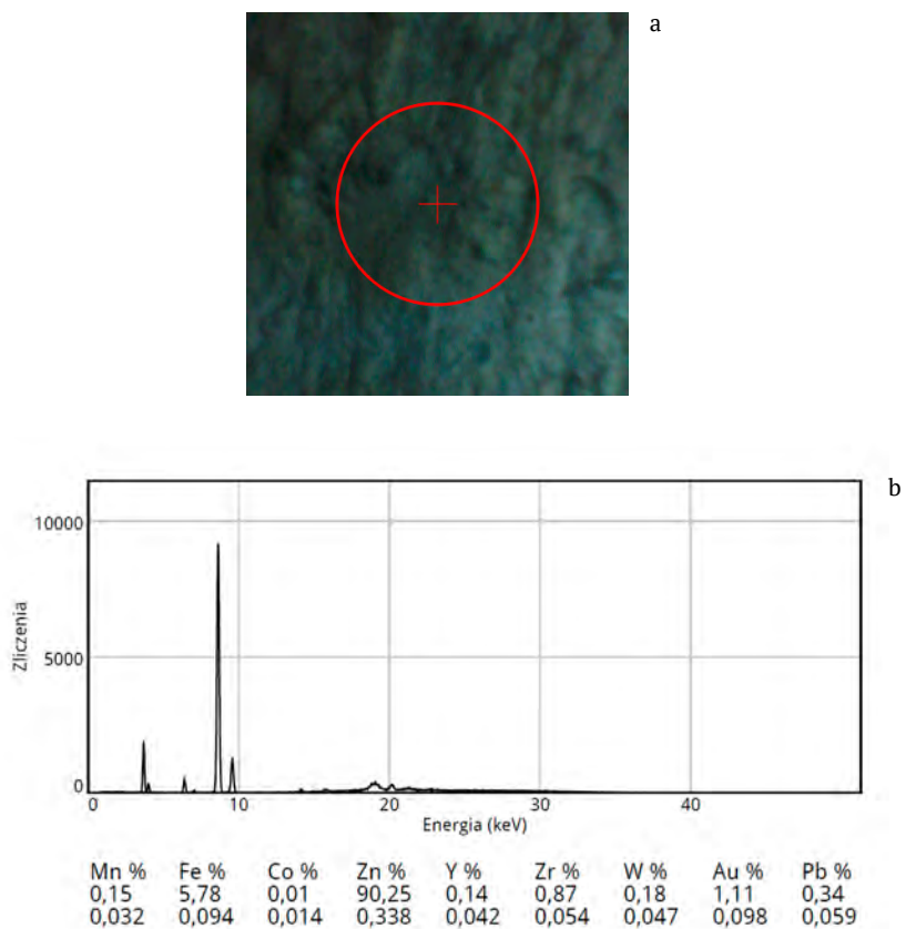
Il. 14. Morąg, kościół św. Apostołów Piotra i Pawła. Prezbiterium, fragment ściany północnej, malowidło Wielka Rodzina Marii . Wyk. J. Raczkowski a – pomiar 2, b – widmo XRF
