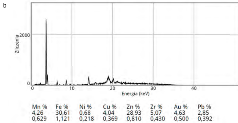
Il. 15. Morąg, kościół św. Apostołów Piotra i Pawła. Prezbiterium, fragment ściany północnej, malowidło Wielka Rodzina Marii . Wyk. J. Raczkowski a – pomiar \beta , b – widmo XRF
