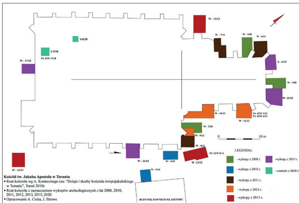
Ryc. 2. Toruń, kościół św. Jakuba. Plan wykopów archeologicznych. Strzałka wskazuje miejsce eksploracji – wykop W-16/15 (oprac. A. Cicha, J. Struwe, W. Miłek)
