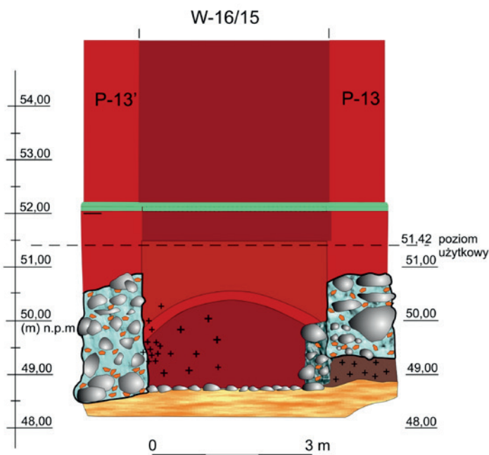
Ryc. 5. Toruń, kościół św. Jakuba. Kaplica św. Walentego – stratyfikacja nawarstwień. Widok na fundamenty i warstwę cmentarną (z krzyżykami) (oprac. K. Sulkowska-Tuszyńska, rys. W. Milek)
