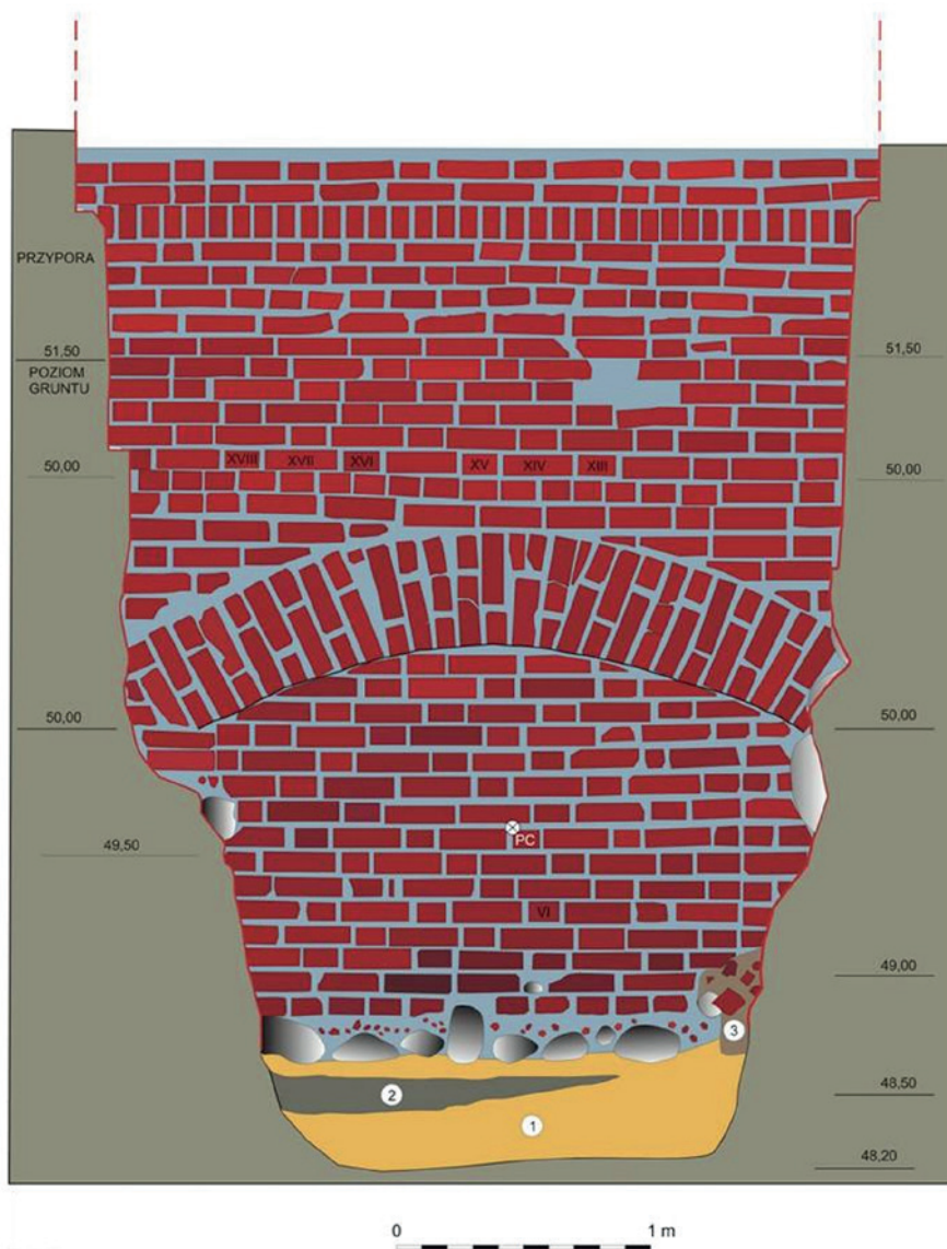
Ryc. 12. Toruń, kościół św. Jakuba. Wykop W-16/15. Widok od południa na fundament i pld. ścianę kaplicy wraz z przekrojem przez przypory. U dołu warstwa spalenizny (rys. M. Magalski, B. Kurtys; oprac. W. Milek)
