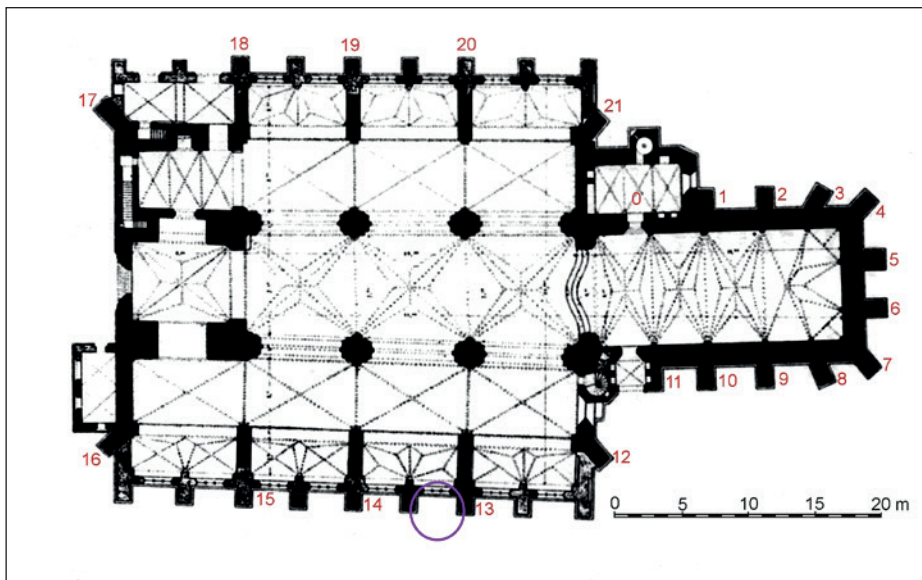
Ryc. 3. Toruń, kościół św. Jakuba. Plan przyziemia kościoła po rozbudowie o kaplice (wg Freymuth 1981, s. 49)
