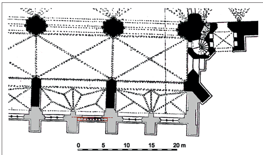
Ryc. 6. Toruń, kościół św. Jakuba. Rzut przyziemia. Zbliżenie na pld. kaplice. Widok od wschodu (wg C. Steinbrecht 1885, tab. VII)
