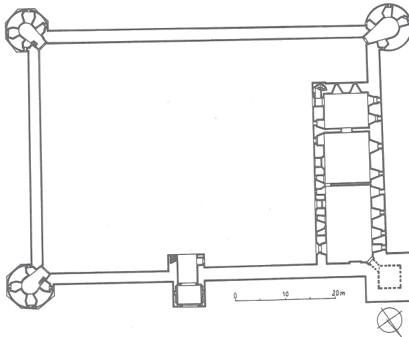
Ryc. 11. Bytów. Rzut zamku, częściowa rekonstrukcja (rys. F. Szymański; Zbiory Fotografii i Rysunków Pomiarowych Instytutu Sztuki PAN, nr inw. RP11164)
