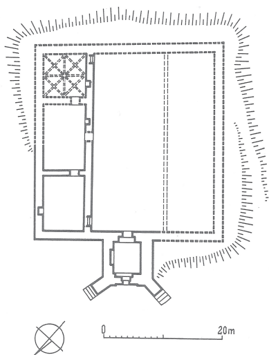
Ryc. 8. Liw. Zamek – rzut budowli w XV–XVI wieku; częściowa rekonstrukcja (rys. R. Kunkel; Zbiory Fotografii i Rysunków Pomiarowych Instytutu Sztuki PAN, nr inw. RP13465)
