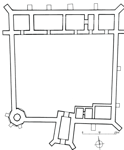
Ryc. 5. Rawa Mazowiecka. Zamek – rzut budowli w XV–XVI wieku; częściowa rekonstrukcja (rys. R. Kunkel; Zbiory Fotografii i Rysunków Pomiarowych Instytutu Sztuki PAN, nr inw. RP14631)
