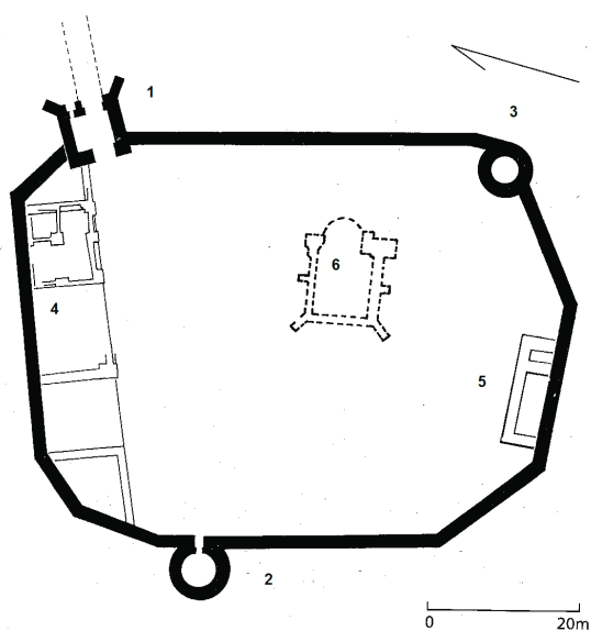
Ryc. 9. Czersk. Rzut ruin zamku (wg Kajzer, Kołodziejcki, Salm 2001)
