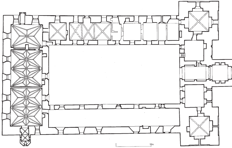
Ryc. 10. Nidzica. Zamek – rzut piętra; częściowa rekonstrukcja (rys. B. Kosińska; Zbiory Fotografii i Rysunków Pomiarowych Instytutu Sztuki PAN, nr inw. RP13691)
