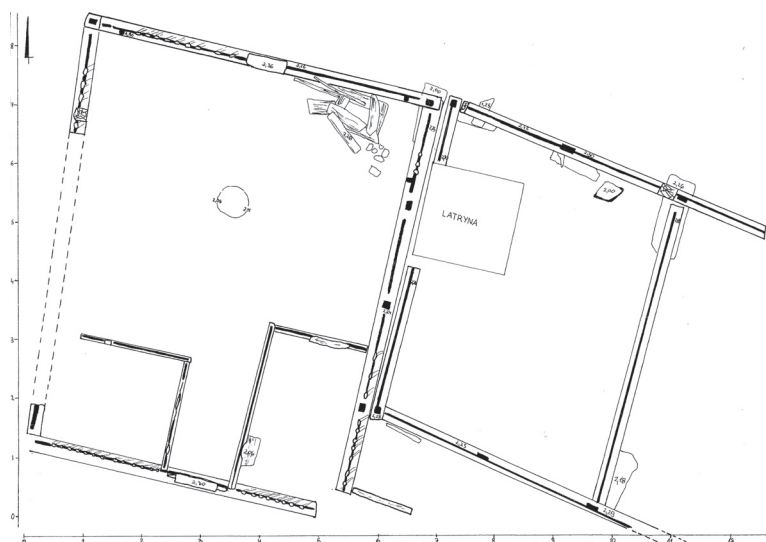
Ryc. 5. Elbląg – Stare Miasto, ul. Tkacka. Plany dwóch budynków o konstrukcji szkieletowej wzniesionych po pożarze miasta, między 1296 a 1304 rokiem (rys. K. Raguze)
