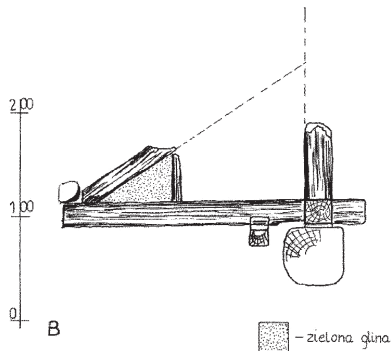
Ryc. 6. Elbląg – Stare Miasto, ul. Rybacka 27. Przekrój ściany wschodniej (A) i północnej (B) budynku o konstrukcji szkieletowej, datowanego między 1270+x/-6 a 1293+8/-6 rokiem (rys. K. Raguze)
